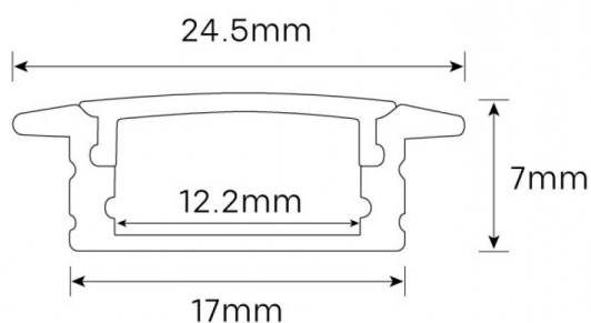
Imagem técnica
